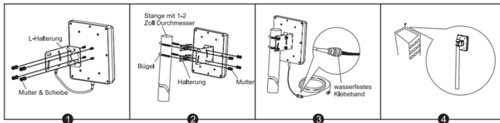
Installation einer Breitband-Außenpanelantenne:
