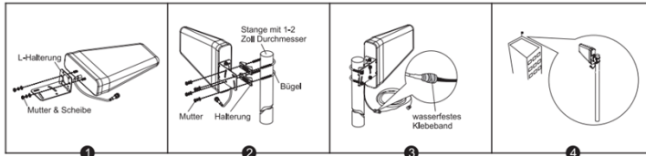
Installation einer Breitband-Außenpanelantenne:
