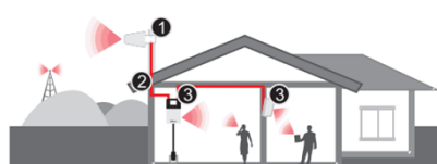
1-Antena direccional de banda ancha para exteriores 2-50pies (15.2m) de cable de baja pérdida HiBoost200 3-Puede agregar una antena interior de panel/omni y 50pies(15.2m) de cable de baja pérdida HiBoost200 para ampliar la cobertura
