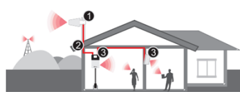
1-Antenna direttiva a banda larga per esterno 2-15,2m Hiboost200 cavo a bassa perdita 3-è possibile aggiungere un'antenna a pannello/omni e 15.2 m Hiboost200 cavo a bassa perdita per estendere la copertura
