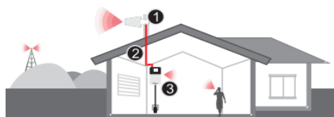
1 - Antenne directionnelle large bande extérieure 2 - Câble Hiboost200 à faible perte de 15,2 m (50 pi) 3 - Amplificateur Hiboost avec antenne intégrée.
