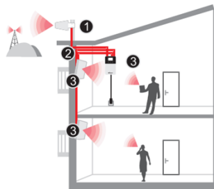
1-Antena direccional de banda ancha para exteriores 2-50pies (15.2m) de cable de baja pérdida HiBoost200 3-Amplificador HiBoost con antena incorporada
