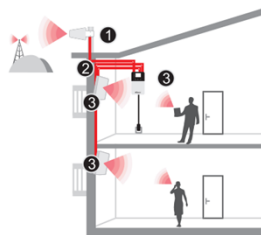
1-Antenna direttiva a banda larga per esterno 2-15,2m Hiboost200 cavo a bassa perdita 3-Amplificatore Hiboost con antenna integrata
