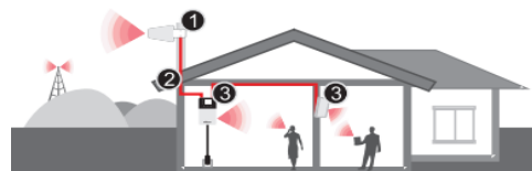
1-Antenne directionnelle large bande extérieure 2-Câble Hiboost200 à faible perte de 15,2 m (50 pi) 3-Y Vous pouvez ajouter un panneau intérieur/antenne omnidirectionnelle et une antenne de 15,2 m (50 pi). Câble Hiboost200 à faible perte pour étendre la couverture
